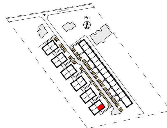
Plan sytuacyjny
